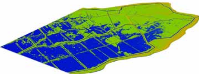
Simulation von Wasserspiegellagen
